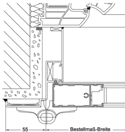
Schnitt seitlich Zargenmontage auf Kunststoff-Fenster
