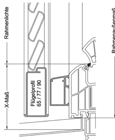
Schnitt unten Grundrahmenmontage auf Kunststoff-Fenster
