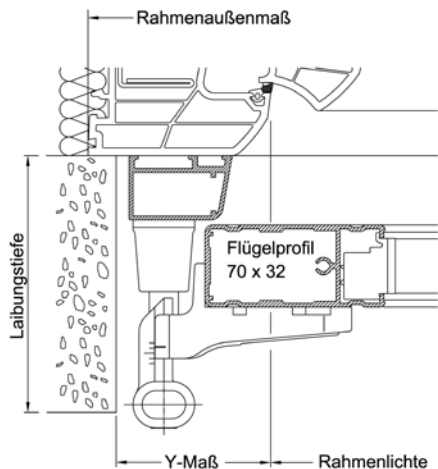
Schnitt seitlich Grundrahmenmontage auf Kunststoff-Fenster
